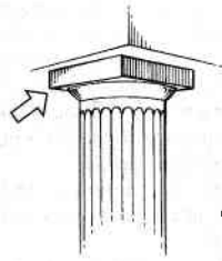
abacă
